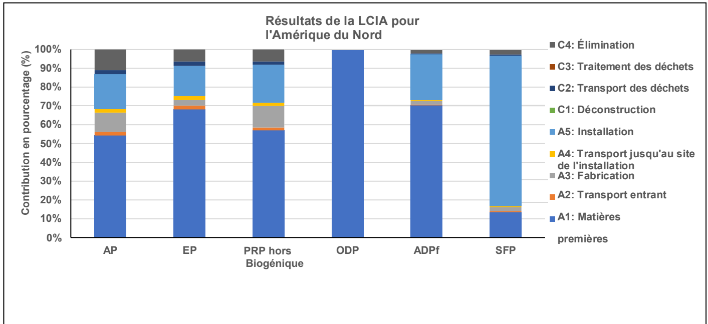
Figure 4 : Analyse de la contribution des résultats du LCIA pour l'Amérique du Nord
